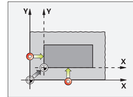
Bezugspunkt setzen z. B. an einer Ecke oder in der Mitte eines Kreisapfens
